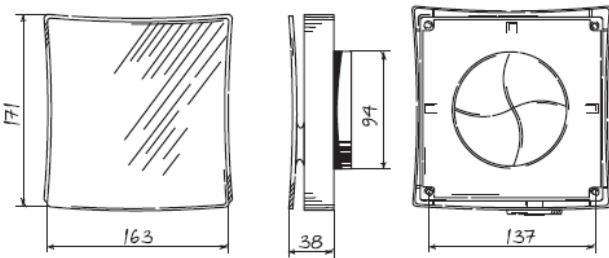
Rejilla externa cuadrada
