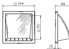
Campana de ventilación de acero inoxidable
