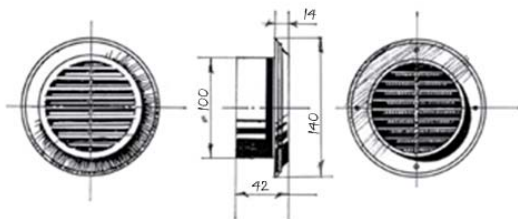
Rejilla externa circular
