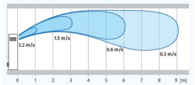
Rango de flujo de aire para el CIVIC EC LB 500
