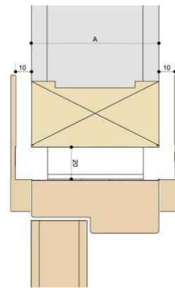
Instalación en puerta normal. Los tapajuntas tienen que ser más gruesos que lo habitual, instalación invertida
